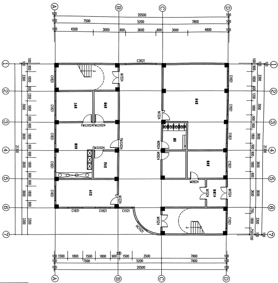
一层平面图 1:100
